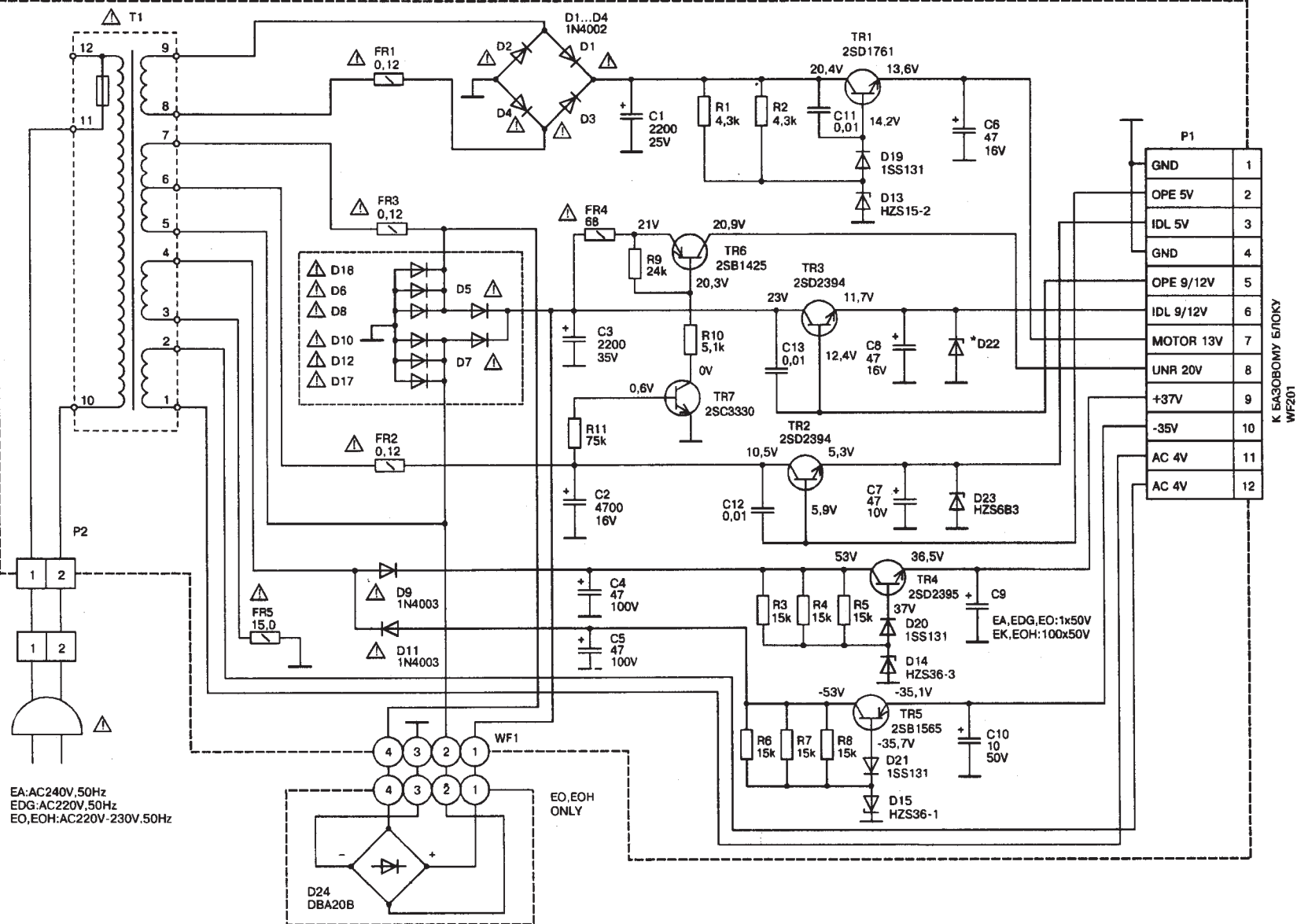
Принципиальная схема источника питания видеомэгнитофонов: VS-G40EA/EDG/EK, VS-G43EK/EOH, VS-G44EK
